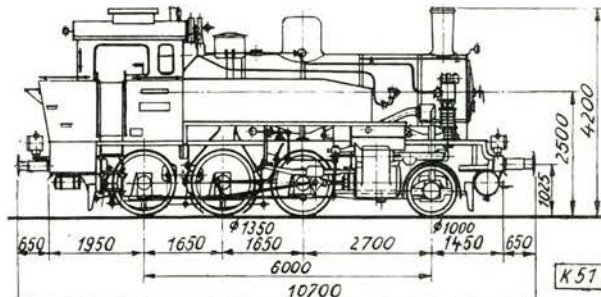
Bild 4 Maßskizze der pr. T 9, spätere Baureihe 91 1-3
