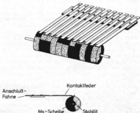
Abb. 6. Schematische Darstellung der in das Märklin-Relais eingesetzten Schaltwalze. Um ein „Hüpfen“ der Kontaktfedern und damit ein Flackern der Ampellämpchen zu vermeiden, sind die kontaktfreien Aussparungen der Ms-Scheiben mit Stabilit express ausgefüllt; danach wird die ganze Walze nochmals überdreht.
