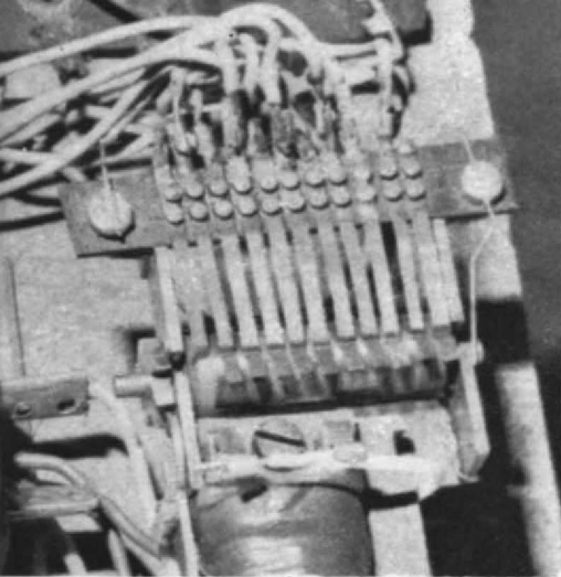
Abb. 3 u. 4. Die gesamte Ampelschaltung, bestehend aus dem abgewandelten Faller-Kontaktschalter, der hier als Phasenschalter fungiert und das Märklin-Umschaltrelais steuert. Dieses steuert seinerseits über die Schaltwalze bzw. die Kontaktfedern (s. Ausschnittsvergrößerung und Abb. 5 u. 6) die verschiedenen Ampellämpchen. Rechts vorn der Gleichrichter (s. Haupttext).
