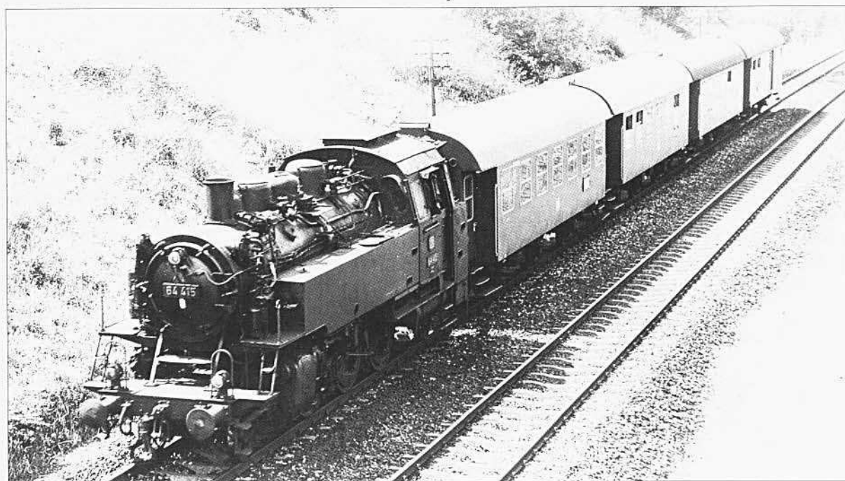
Bild 7 (oben): Die Preußischen Staatsbahnen setzten auf die Achsfolge 1' C, um – wie hier 1940 mit der 74 1201 in Berlin – den Vorortverkehr zu bewältigen. Abb.: C. Bellingrodt, Sammlung Merker-Verlag
