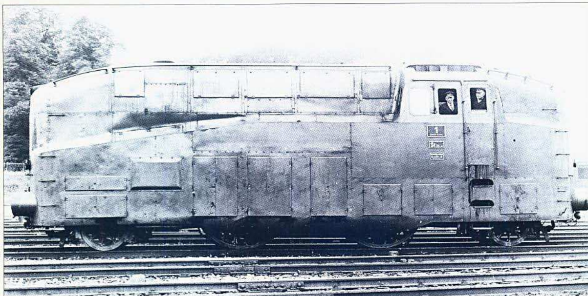
Bild 10: Aus der LBE-Nr. 1 wurde nach der Übernahme durch die DRG 1937 die Lokomotive 60 001.
