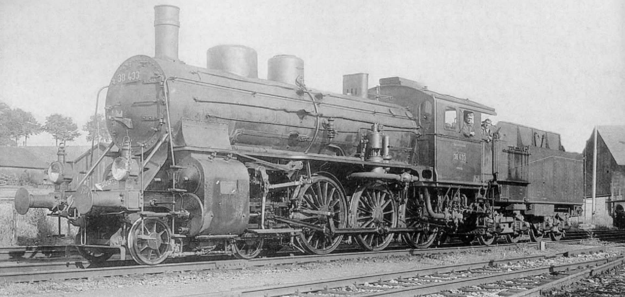
Abb. 26. Das bayerische Pendant zur preußischen P 8 stellt die P3/5H dar, die allerdings – gemäß Maffei'scher Lokbau-Tradition – ein Vierzylinder-Verbund-Triebwerk aufwies.
