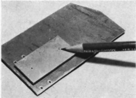
Abb. 5. Untersicht der Weiche. Die Zungen sind aus einer als Extra-Teil eingesetzten dickeren Platte herausgefräst. Der Bleistift deutet auf den Drehpunkt dieser Platte, gegenüber liegt die Bohrung für den Stelldraht. Zur Schmierung der beweglichen Weichteile empfiehlt der Hersteller „La Beille 101“ (z. B. von Old Pullman erhältlich).
