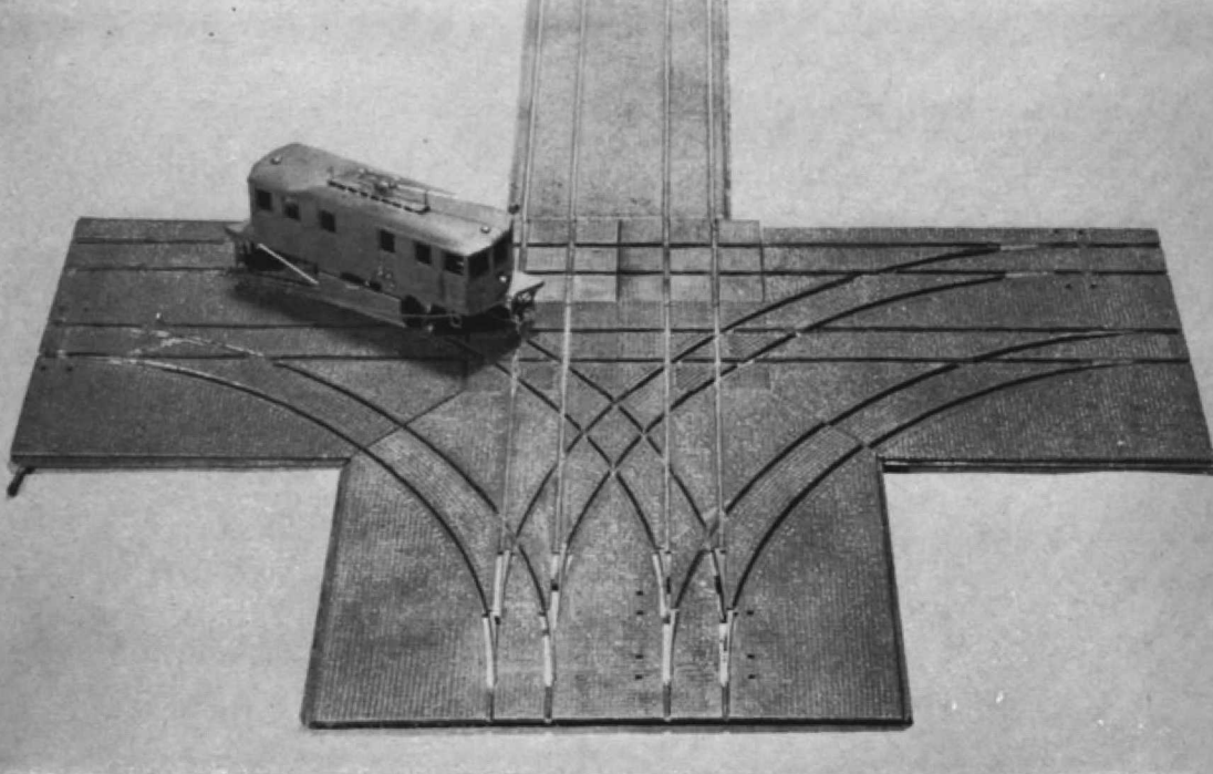
Abb. 1 u. 2. Eine Kreuzung samt Abzweigung von zwei zweigleisigen Strecken, gebildet aus den Strab-Gleiselementen von Lindtram. Abb. 2 verdeutlicht, aus welchen Elementen (insgesamt 8) diese komplizierte Figur zusammengesetzt wurde. Das Strab-Modell stammt übrigens von Fairfield und stellt einen Dienstwagen mit Kehrbürsten dar (US-Vorbild).
