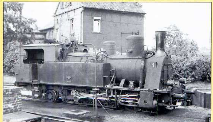
Bild 19: Bei der Hafenbahn Hamm war sie 1961 noch die Nummer 1. Aus verschiedenen Details läßt sich auf eine Esslinger T 26 schließen. Abb.: Sammlung Grundmann
