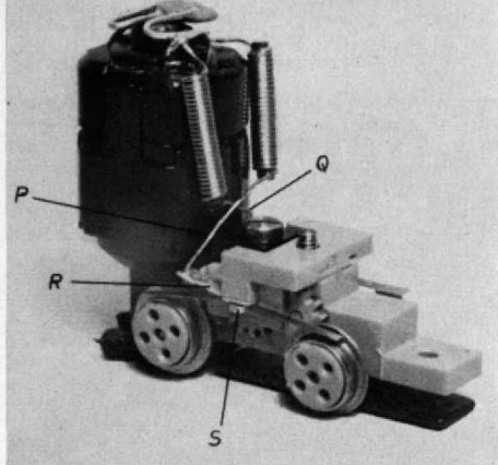
Abb. 9. Hier ist die Umpolung bei dem Egger-Chassis bereits erfolgt: die beiden Anschlüsse P und Q verlaufen überkreuz. Wie im Text zu Abb. 8 bereits gesagt, müssen auch die Kontaktbleche R mit umgewechselt werden. Nach dem Lösen der kleinen Schraube S können sie abgenommen werden.
