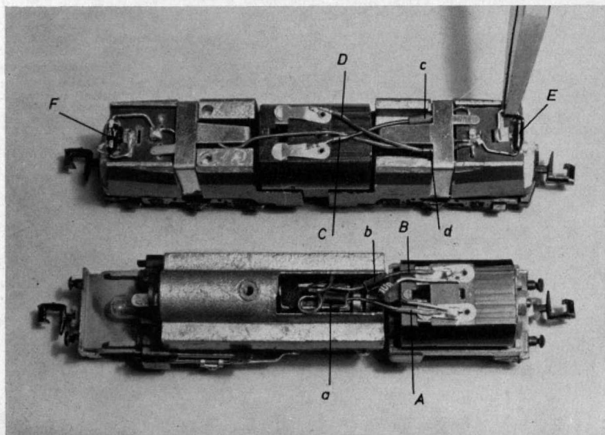
Abb. 2. Die gleichen Lok-Chassis wie in Abb. 1, jedoch nach dem Umpolen. Die Buchstabenbezeichnungen entsprechen denen der Abb. 1. Bei dem Chassis der BR 66 erkennt man im Vergleich zu Abb. 1 an den Ferritröhrchen, daß beide Zuleitungen vertauscht wurden, beim E10-Chassis sind die Zuleitungen überkreuz gelegt.
