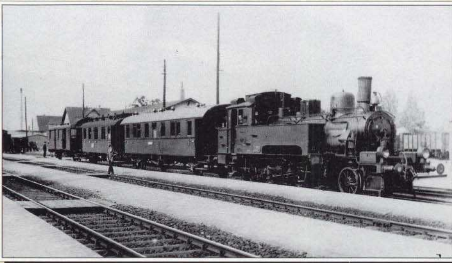
Bild 7 (oben links): Im Bahnhof Beucha wartet eine 71 er mit einem kleinen Personenzug auf die Weiterfahrt.
