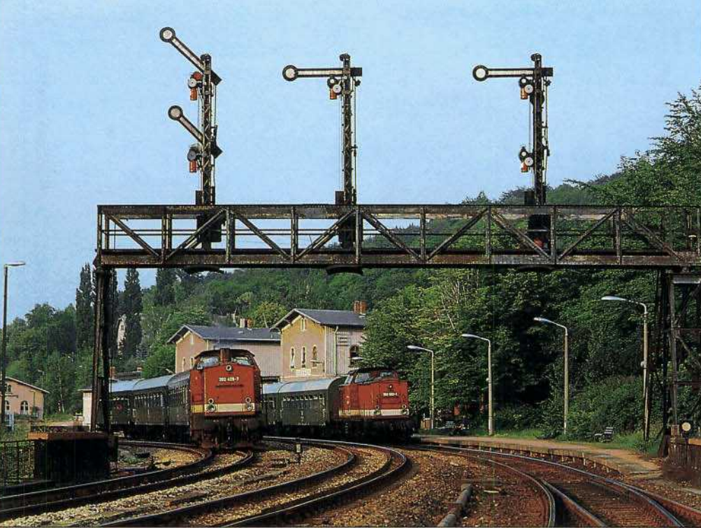
Bild 16: Roßwein am 26. August 1993. Auf der Signalbrücke zeigt das Signal für das Gleis nach Leipzig Hp 2 für den P 7448. Rechts wartet P 8961 mit dem Zug nach Niederwiesa.
