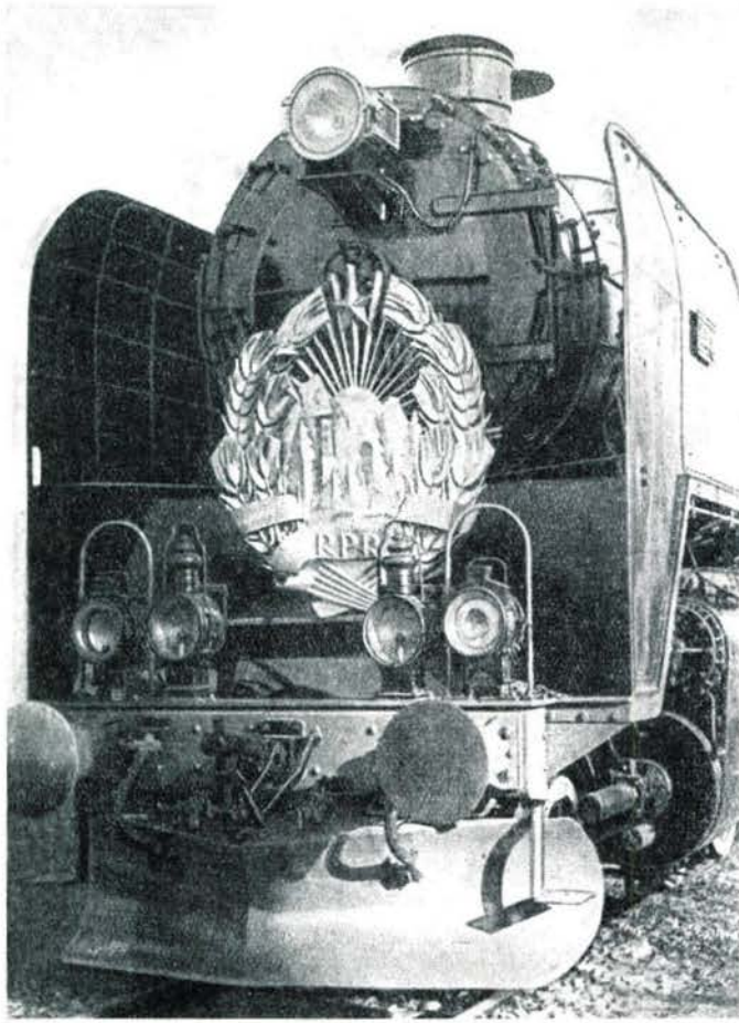
Stirnansicht einer schweren Güterzuglokomotive, Achsfolge 1'E, aus der Volksrepublik Rumänien
