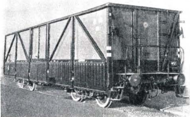
Die Bilder in der linken Spalte zeigen einen G-, einen GG- und einen OO-Wagen aus der Rumänischen Volksrepublik. Der vierachsige offene Güterwagen ist mit seitlicher Selbstentladeeinrichtung versehen. Bilder in der rechten Spalte von oben nach unten: Vierachsiger Schnellzugwagen (Schlafwagen) mit geschlossenen Übergängen durch Faltenbälge aus der Volksrepublik Polen
