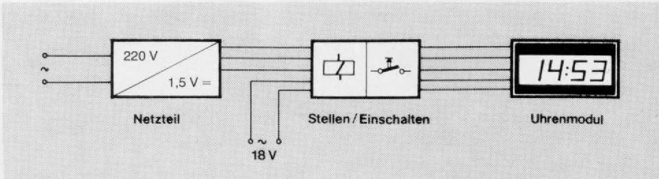
Abb. 1. Das Blockschaltbild von Stromversorgung, Einstellautomatik und Uhrenmodul.
