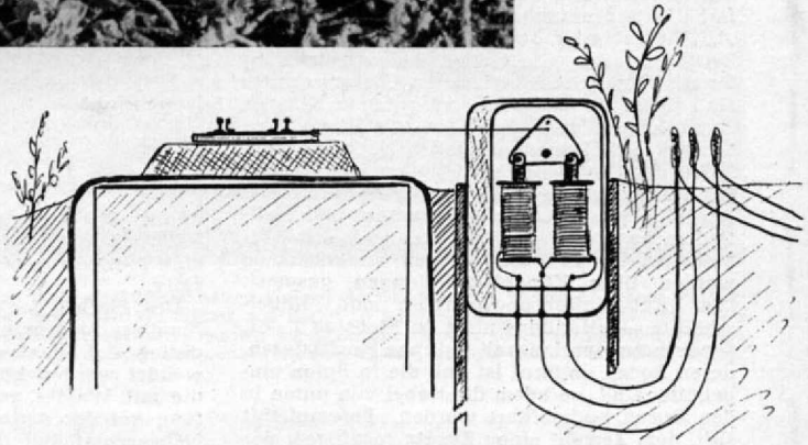
Abb. 4. Schemazeichnung für den Einbau der Weichenantriebe. Nähere Erläuterungen siehe Text. Es müssen unbedingt die Redlin-Antriebe verwendet werden. Andere gute Fabrikate erfüllen ihren Zweck genauso.
