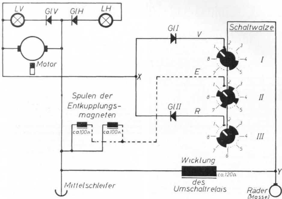
Abb. 1. Nicht nur zur bildlichen Erläuterung des Textes, sondern auch als Arbeitsvorlage beim Umschalten einer Gleichstromlokomotive auf Wechselstrombetrieb soll dieses Schaltschema dienen. Wir haben hier – abweichend von der Abbildung in Heft 16/XII, S. 645 – die Schaltwalze anders gezeichnet, weil wir meinen, daß diese Darstellung anschaulicher ist als die normgerechte. Die drei Kontaktscheiben I, II und III der Schaltwalze sind massführend und auf gemeinsamer Achse angebracht. Bei jedem Überspannungsimpuls bewegen sich die Kontaktscheiben im Uhrzeigersinn um einen Schritt weiter und schalten damit wahlweise die Fahrtrichtung der Lok um bzw. die Entkupplungsmagneten ein oder aus. Als Gleichrichter finden solche für Einwegschaltung Verwendung; je nach Stromverbrauch des Motors können unterschiedliche Ventilzellen (Gleichrichter) eingebaut werden. Für GI I und GI II z. B. Conrad LC 1350. GI V und GI H sind in der Regel bereits vorhanden, es sei denn, es handelt sich um einen Totalumbau. Der Stromverbrauch der Lok erhöht sich bei 12 V = um etwa 0,1 Amp. Die eingeschaltete Entkupplung verbraucht bei 8 V = ca. 160 mA zusätzlich.
