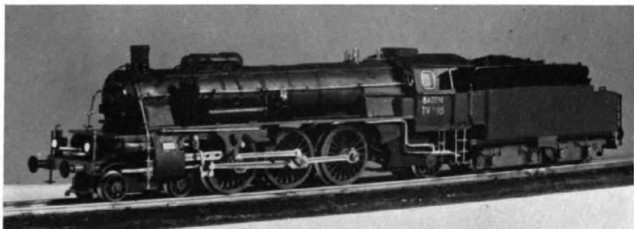
Abb. 2. Das „neueste“ der innerhalb von 10 Jahren entstandenen 14 selbstgebauten Modelle: die „18“ (ehemalige bad. IV h) in H0-Größe, mit einem kräftigen MÄRKLIN-Motor und (vorrätigen) HELLER-Rädern.
