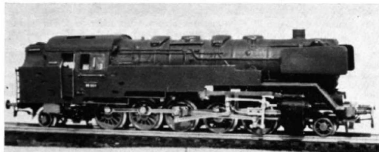
Abb. 8. Aus der MÄRKLIN BR 44 entstand diese 1'E1'-h 3-Gt der BR 85 und beweist wieder einmal mehr, daß unter Verwendung von Fertigteilen durchaus gute und beste Modelle anderer Type zustandekommen können!
