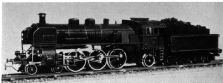
Abb. 6. Bayr S 3/6 (BR 18 1 ), unter Verwendung von MÄRKLIN-Rädern und -Motor. Kessel, Räder und Tenderseitenteile grün, Rahmen, Tenderdrehgestelle und Rauchkammertür schwarz.
