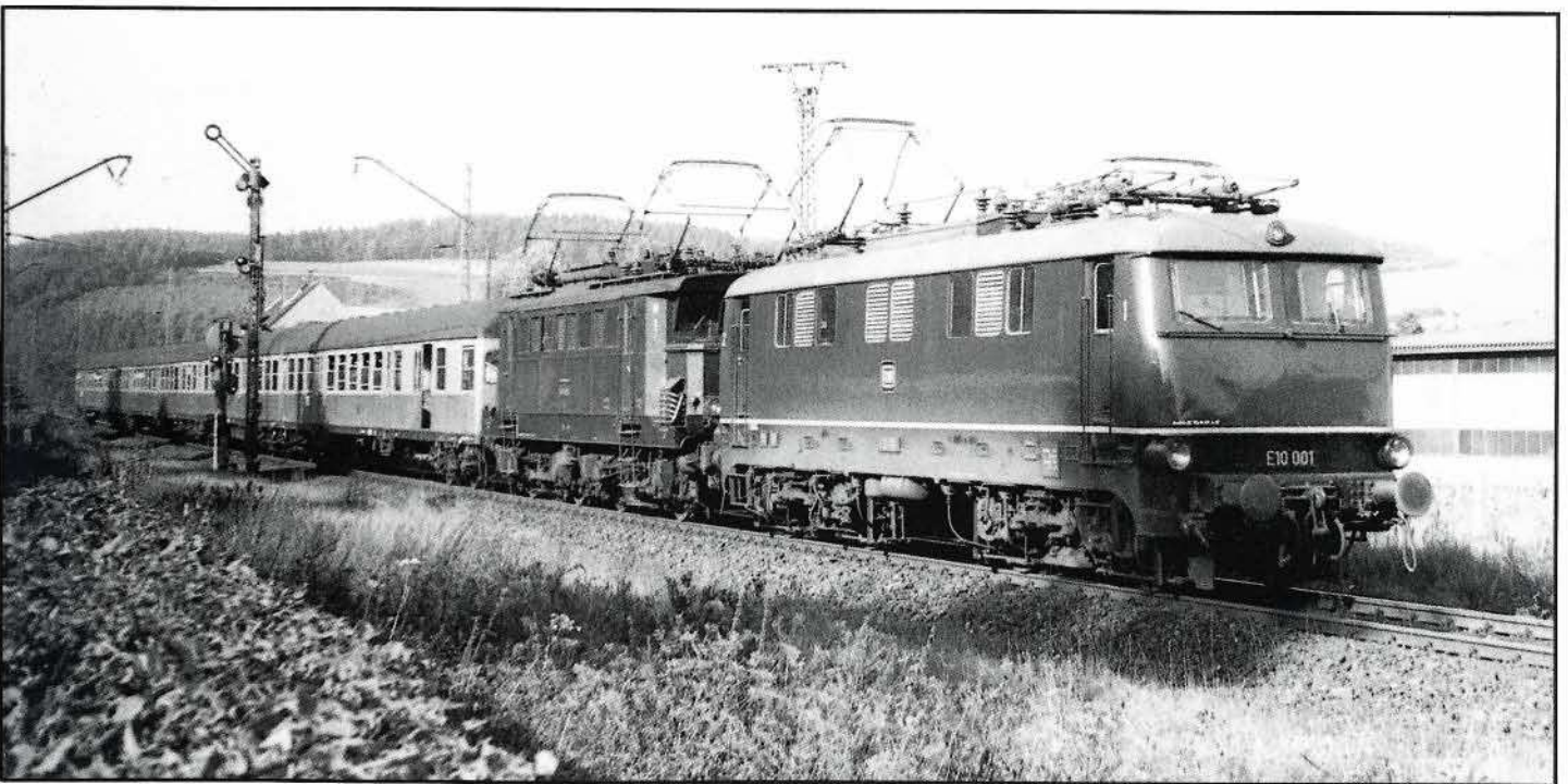
Bild 10: Die E 10 001 (Bw Nürnberg Hbf) als Leervorspann vor der E 44 107 (Bw Nürnberg Hbf) mit einem Personenzug zwischen Kronach und Neuses am 26. September 1967. Abb.: Dr. G. Scheingraber
