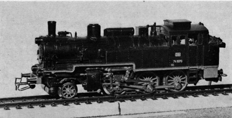
Abb. 139. Die 74 1070 nochmals aus anderer Sicht, bei der das Charakteristische dieser Loktype deutlicher in Erscheinung tritt. Die Zylinderblöcke dürften etwas voluminöser (als bei der „24“) sein (wodurch die Lücke zwischen Lauftrad und Zylinderblock zum Verschwinden käme), aber wir wollen nicht päpstlicher sein . . .
