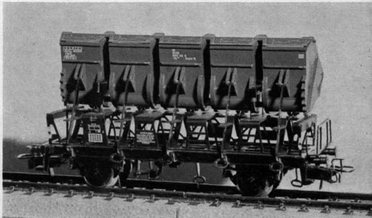
Abb. 142. Dasselbe Modell, von der anderen Seite gesehen. Nach Ausrasten der mittleren Haltestange sind sämtliche Mulden kippar.
