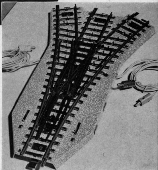
Abb. 149. Die symmetrische Dreiwegweiche (ohne Weichenlaternen) – nah besehen.
