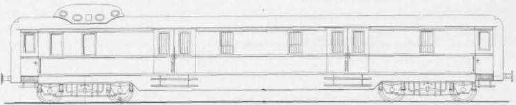
Abb. 17. Gleichfalls als Liliput-Modell zu erwarten: der AB 4ü der DB (ex BC 4ü oder ABC 4ü-39). Hier die Abteilseite eines nach UIC-Norm beschrifteten DB-Wagens. Dieser Wagen und der der Abb. 15 haben übrigens Dachlüfter der Bauart „Wendler“, während der Schürzenwagen der Abb. 18 mit „Kuckuck“-Luftsaugern ausgerüstet ist. Beide Arten waren anzutreffen. (Foto: Europa-Waggonarchiv Willke, Stuttgart)
