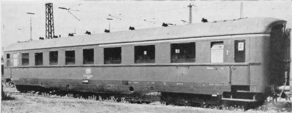
Abb. 17. Gleichfalls als Liliput-Modell zu erwarten: der AB 4ü der DB (ex BC 4ü oder ABC 4ü-39). Hier die Abteilseite eines nach UIC-Norm beschrifteten DB-Wagens. Dieser Wagen und der der Abb. 15 haben übrigens Dachlüfter der Bauart „Wendler“, während der Schürzenwagen der Abb. 18 mit „Kuckuck“-Luftsaugern ausgerüstet ist. Beide Arten waren anzutreffen. (Foto: Europa-Waggonarchiv Willke, Stuttgart)
