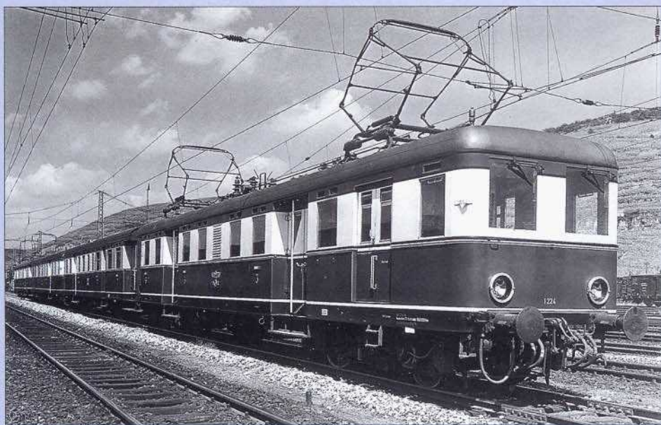
Robust: ET 65 mit zwei Zwischenwagen. Aufnahme um 1939. Abb.: Sammlung Messerschmidt
