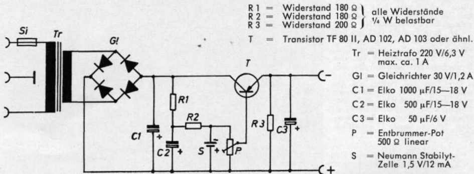
Abb. 1. Schaltschema und Stückliste für das elektronisch stabilisierte Netzgerät.
