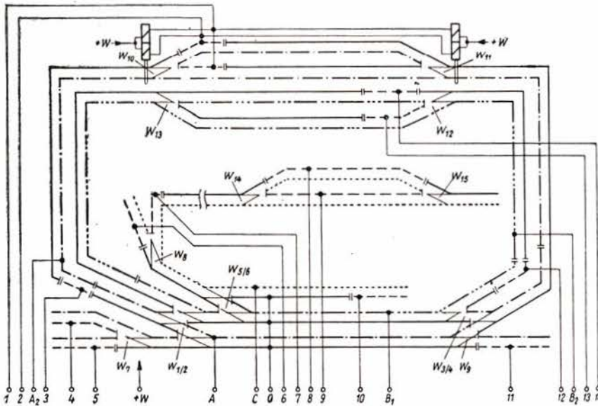
Bild 1 Schaltung der Modelleisenbahnanlage Altenberg—Holzungen—Wiesmar. Die Schaltung der Weichen ist nur für W 10 und W 11 angegeben, um eine bessere Übersicht zu gewährleisten. In den Weichen und bei den abschaltbaren Gleisstücken sind die Leitungen gleicher Kennzeichnung miteinander verbunden.
