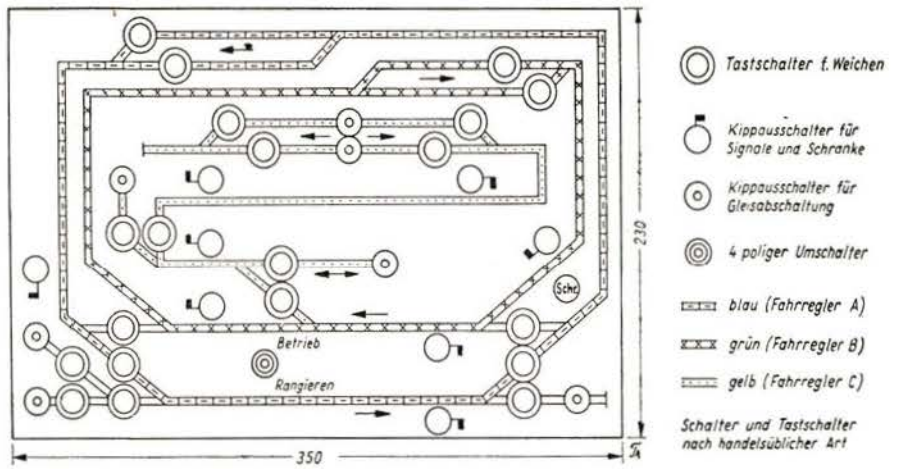
Bild 3 Das Gleisbildstellwerk veranschaulicht die Modelleisenbahnanlage in vereinfachter Form. Dadurch, daß jeder Schalter und jede Taste an der entsprechenden Stelle sitzt, ist die Bedienung sehr übersichtlich und einfach.
