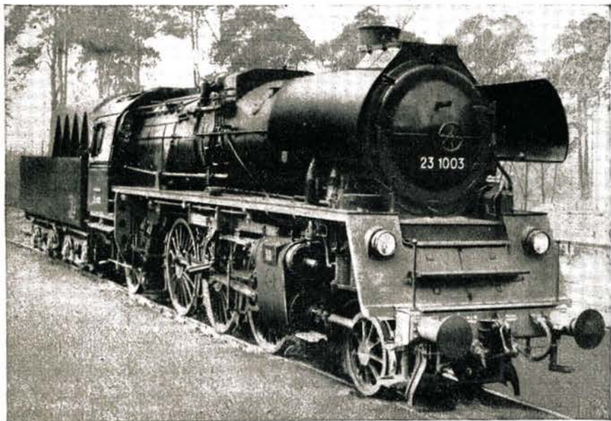
Unser Bild zeigt die Neubau-Personenzuglokomotive der Baureihe 23 10 . Die Lokomotive 23 1003 unterscheidet sich infolge einiger baulicher Veränderungen von den ersten Lokomotiven 23 1001 und 1002 dieser Baureihe.
