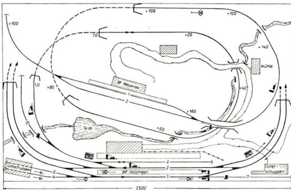
Bild 4 Gleisplan der Modelleisenbahnanlage Altenberg—Holzlingen—Wiesmar aus Heft 1/57.
