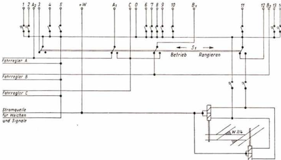
Bild 2 Schaltung im Bedienungsfeld der Anlage ohne Signale und Weichen. Rechts unten die Schaltung der Weichen W 3/4, (die Weichen W 1/2 und 5/6 werden sinngemäß geschaltet). Die Besonderheit liegt darin, daß die Zuleitung über den Umschalter führt, eine Gleisverbindung also nur in Stellung „Rangieren“ möglich ist.
