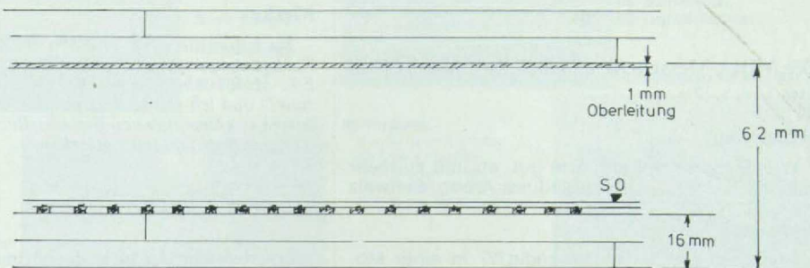
Abb. 4. Nach diesen Einbaumaßen sollte man sich richten, wenn man eine Oberleitung in die Wendel einbauen möchte (Abbildungsmaßstab 1:2).
