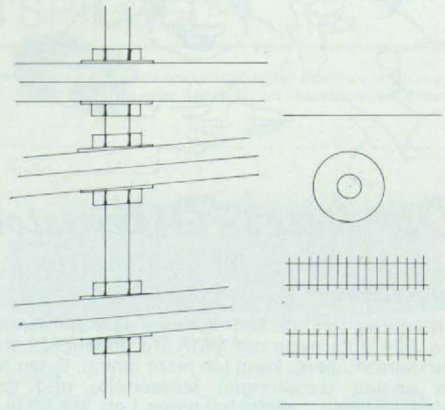
Abb. 3. Mit den (hier schematisch dargestellten) Gewindestangen lassen sich die einzelnen Ebenen justieren; rechts die Draufsicht.
