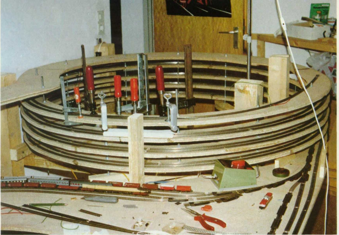
Abb. 1. Mit Schraubzwingen werden die einzelnen Spanplatten-Segmente zusammengepreßt, bis der Holzleim abge- bunden hat. Die vier Kanthölzer ergeben das stabile Grundgerüst.
