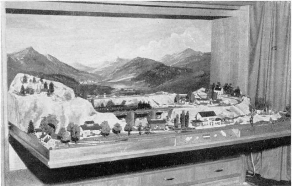
Abb. 4-6. Der Modellbahnschrank, geöffnet und geschlossen und Rahmendetail
