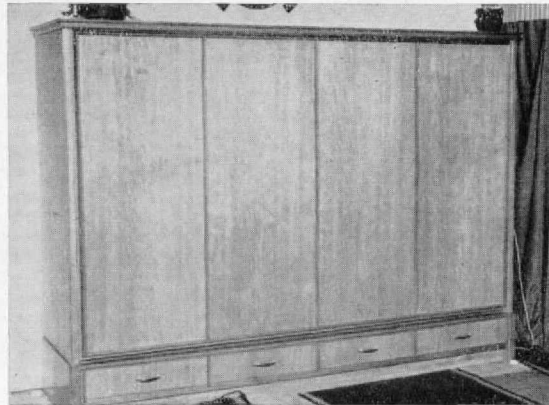
Abb. 4-6. Der Modellbahnschrank, geöffnet und geschlossen und Rahmendetail
