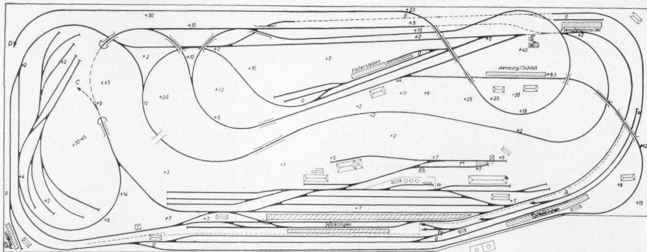
↑ Abb. 4. Gleisplan der Anlage des Herrn Großhans, Neu-Isenburg. Zeichnung im Maßstab 1:40. Größe der Anlage: 7x2,65 m. Beim Aufbau dieser recht großen Anlage fanden ausschließlich Märklin-Punktcontactgleise Verwendung. Der sanft gebogene Gleisbogen in der Mitte der Anlage wurde nur aus geraden Gleisen, die jeweils ganz wenig abgelenkt wurden, zusammengesetzt, während sich die Gleisstücke des Spitalkirchner Bogens (im Gleisplan in der rechten unteren Ecke) einer besonderen Behandlung „erfreuten“: 15
