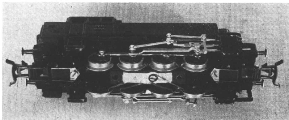
Abb. 5. Radschleifer aus Bronzefederdraht bei einer mehrachsigen Lok (hier BR 81).
