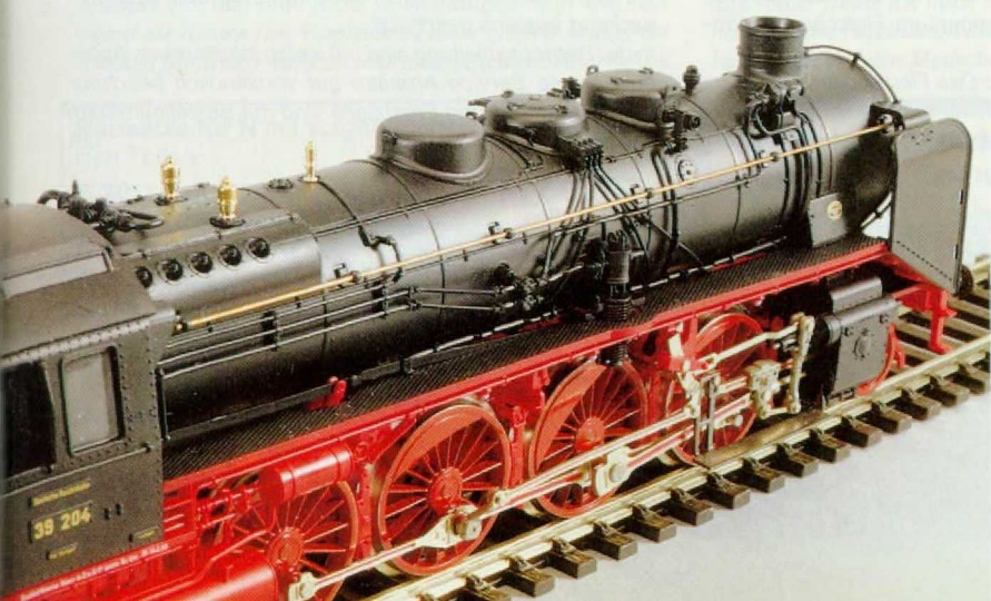
Bild 2. Dampflok-Armaturen vom Feinsten – wer mag da noch „supern“? Die Kardangelenke der Anstellstangen (Bildmitte) stehen je verschieden, als ob der Lokführer gerade an ihnen gedreht hätte. Eingesetzte Sandrohre, Dampf- und Wasserleitungen – darüber braucht man schon gar nicht mehr zu reden.
