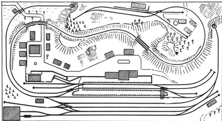
Plan 10 Maßstab 1 : 25 – Anlagengröße 2,80 x 1,50 m Ein Bahnhof mit sehr gut wirkenden Weichenstraßen – wie geschaffen für einen Gleisselbstbauer! Der Bahnhofsbetrieb ist Hauptzweck, die Nebenbahn eine nette Zugabe. Es ist empfehlenswert, unter dem Hügel einen Einsatz- und Ausweichbahnhof zu schaffen, um den Hauptbahnhof mit den nötigen Zügen abwechselnd „füttern“ zu können!
