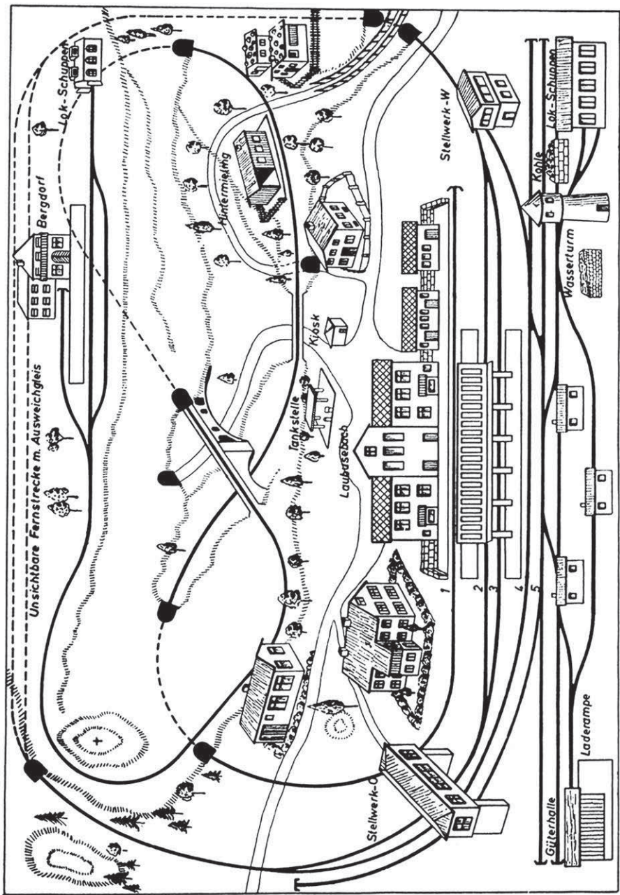
Plan 4 Maßstab 1 : 18 — Anlagengröße 3,00 x 2,00 m. Eine eingeleisige Strecke mit (getrennter) Nebenbahn ins Gebirge. Eine Verbindung zur Hauptbahn ist jedoch leicht zu schaffen.
