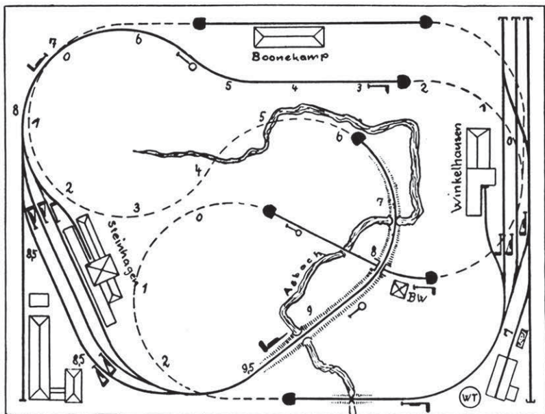
Plan 9 Maßstab 1 : 20 – Anlagengröße ca. 2,00 x 1,50 m Lassen Sie sich durch die „Schleifen“ nicht irritieren, sie treten überhaupt nicht in Erscheinung und wirken sich betrieblich nur günstig aus (Fahrzeitverlängerung).
