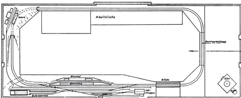
Plan 5 Maßstab 1 : 55 – Anlagengröße 6,00 x 2,70 m – eigentlich eine in einem ausrangierten Waggon eingebaute Clubanlage (Wolfenbüttel), enthält jedoch eine Durchgangsstation, die beispielhaft ist und genügend Platz (z. B. auf einem Dachboden) gut als Vorlage dienen kann.
