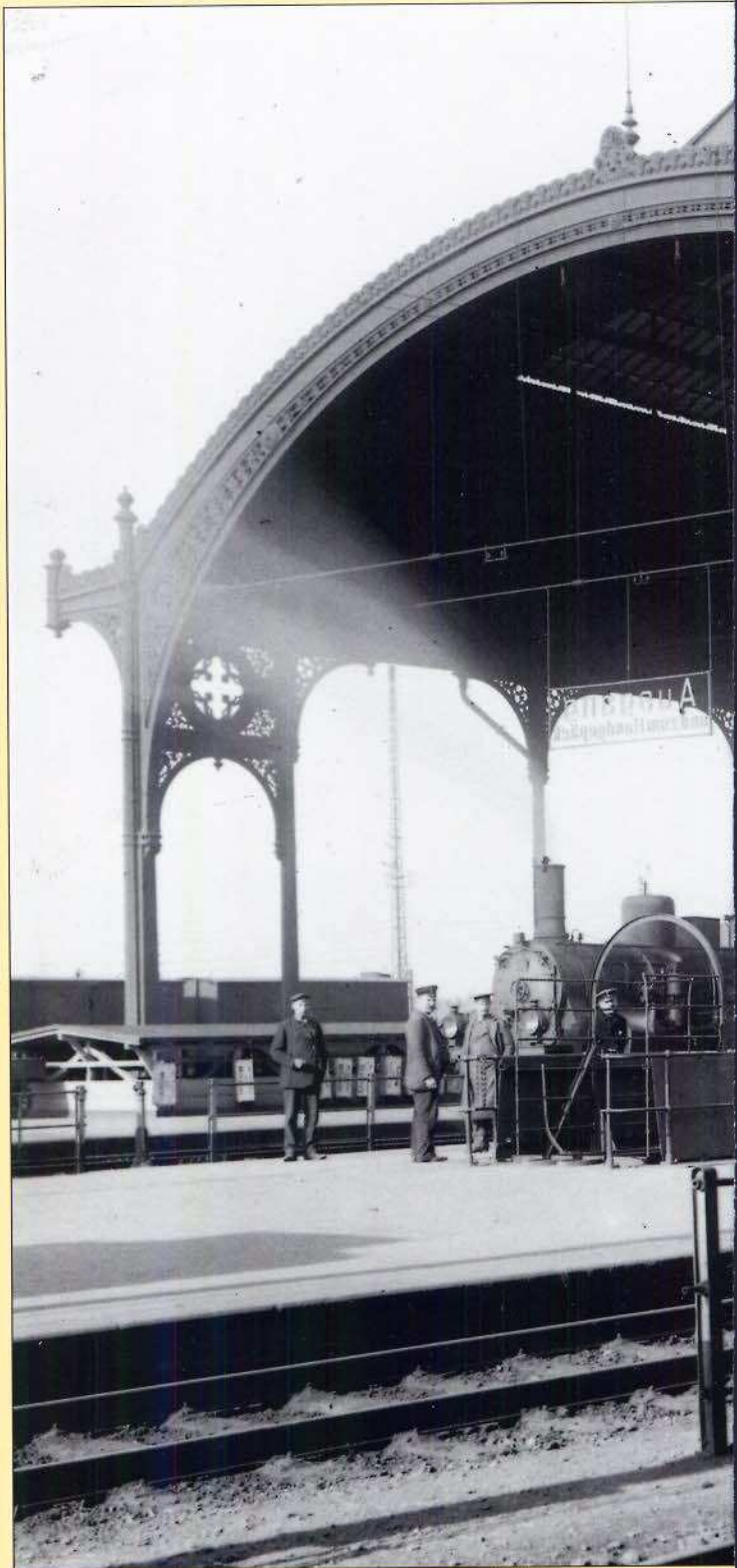
Bild 6: Unmittelbar vor den Hallen des Straßburger Bahnhofs befanden sich Schiebebühnen zum platzsparenden Umsetzen von Loks und Wagen. Nicht nur die Fahrzeuge, auch die Signale sehen "typisch preußisch" aus. Fotos 4 bis 6: Deutsches Museum, Sammlung Klee
