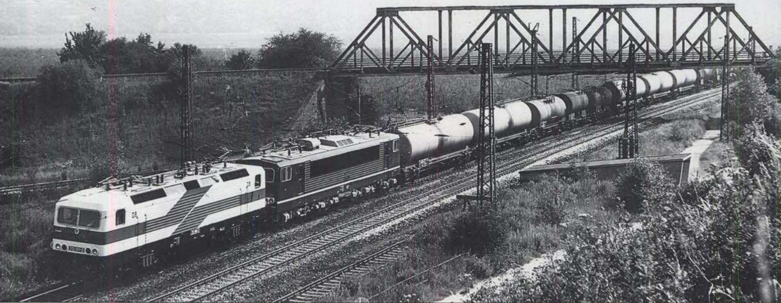
Bild 5: Die Baumusterlokomotive 212 001 wurde auch im Güterzugdienst erprobt. Am 10. Juli 1982 zieht sie hier auf der Strecke Leipzig – Großkorbetha einen Kesselwagen-Ganzzug (und eine abgebügelte Lokomotive der Baureihe 250). Foto: M. Malke
