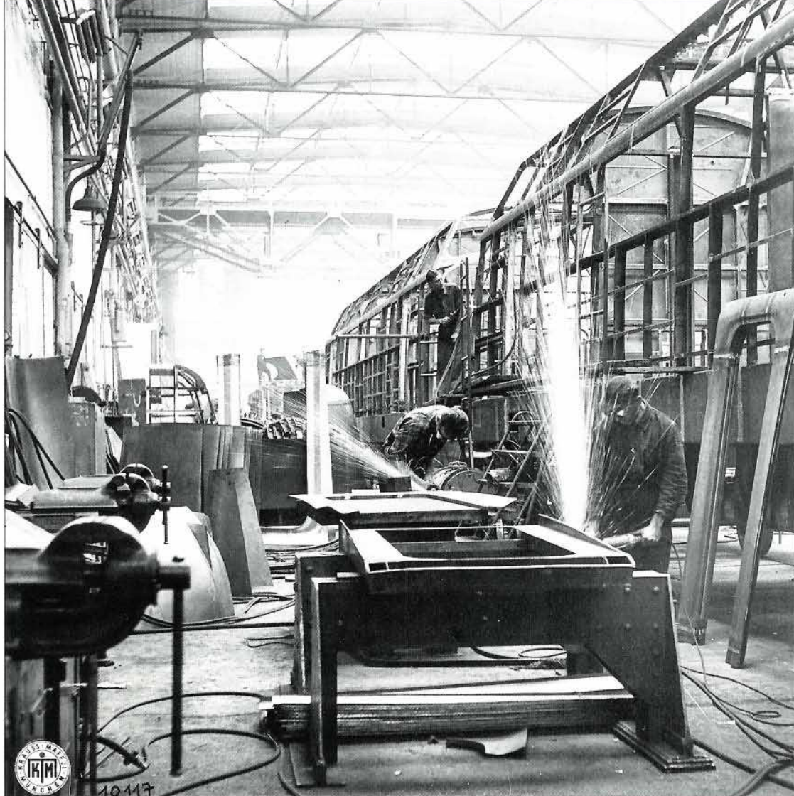
Bild 9: V 200-Drehgestell; dahinter Laufwerk und fertige Lokomotiven der Baureihe 65 sowie ein S 3/6-Neubaukessel. Werkfoto Krauss-Maffei
