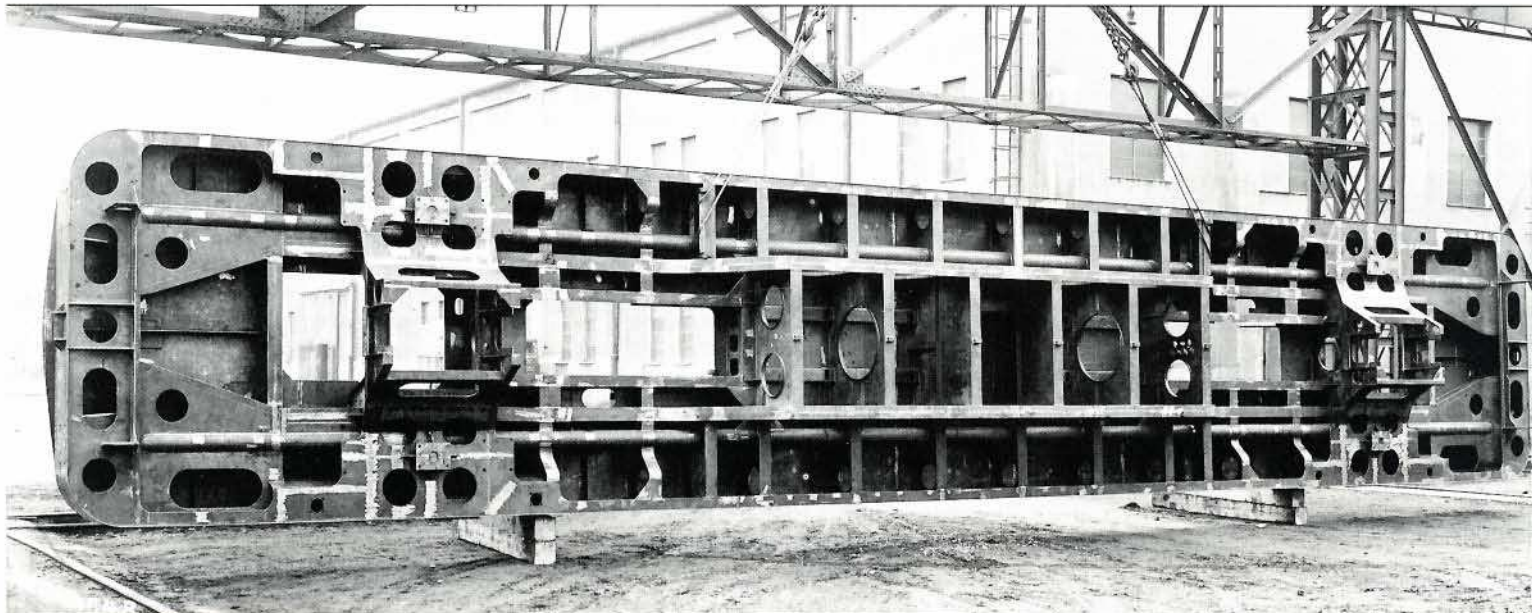
Bild 6: V 200-Rahmen von unten. Werkfoto Krauss-Maffei
