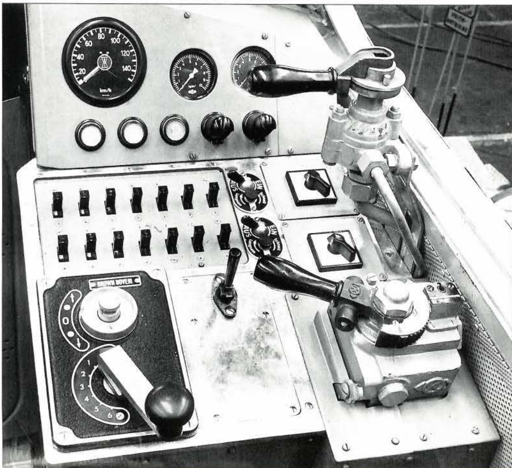
Bild 15: Führerpult der ersten Bauserie (V 200 006 bis 055). Werkfoto Krauss-Maffei
