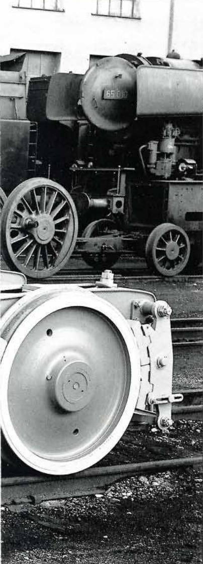
Bild 9: V 200-Drehgestell; dahinter Laufwerk und fertige Lokomotiven der Baureihe 65 sowie ein S 3/6-Neubaukessel. Werkfoto Krauss-Maffei
