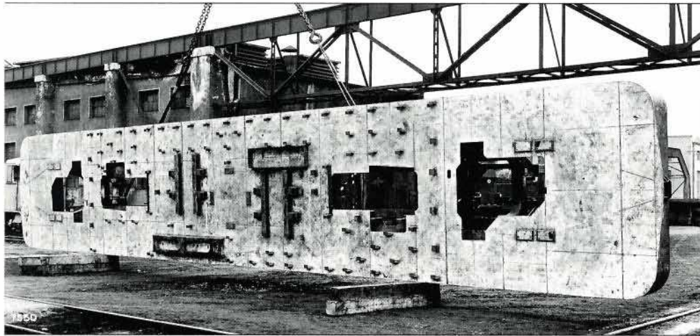
Bild 5: Geschweißter Rahmen der Baureihe V 200 von oben mit den Ausschnitten für die Mekydro-Getriebe und die Dieselmotoren. Werkfoto Krauss-Maffei
