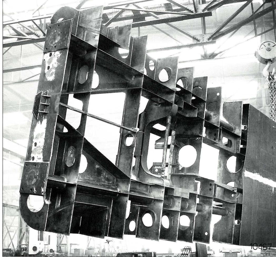
Bild 7 (oben rechts): Rahmen in der Fertigung: Gut zu erkennen sind die beiden durchlaufenden Rohre, auf die die Querverbindungen "aufgefädelt" werden. Werkfoto Krauss-Maffei
