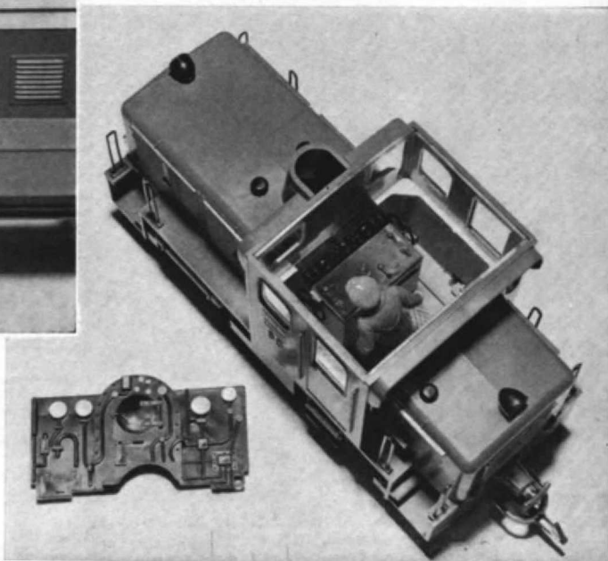
Abb. 5. Auch die LGB-Loks weisen fein detaillierte Inneneinrichtungen auf und der Fahrer steht bei der Diesellok 2060 erfreulicherweise mal hinterm Fahrpult. Links eine Kesselarmaturen-Attrappe der LGB-Loks 1, 2 u. 4.
