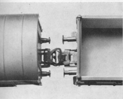
Abb. 1. Vergleichsaufnahme: Links Märklinwagen mit fabrikmäßigen Puffern, rechts mit maßstäblich richtigen Federpuffern.
