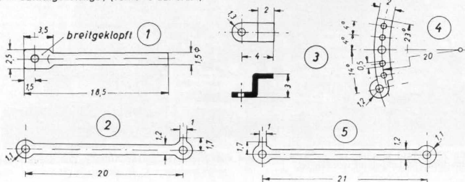
Abb. 6. Die Steuerungssteile im Maßstab 2:1. Alle nicht vermaßten Bohrungen haben 1 mm Ø. 1 = Schieberstange (Ns 1,5 mm Ø), 2 = Schieberschubstange, 3 = Schwingenlager, 4 = Schwinde, 5 = Schwingenstange; (Teil 6—8 auf S. 291).
