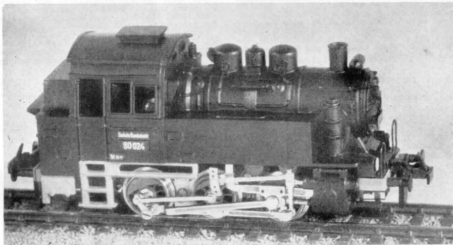
Abb. 3. Vorbild und Muster — eine „751“, die vom Verfasser dieses Artikels zum Modell der Bauartreihe 80 umgebaut worden ist.
