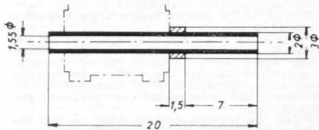
Abb. 8. Kolbenstangenschutzrohr mit der Nachbildung der vorderen Kolbenstangenentrags- bzw. Stoffbuchse. Die gestrichelte Linie deutet die Zylinderumgrenzung an (Maßstab 2:1).
