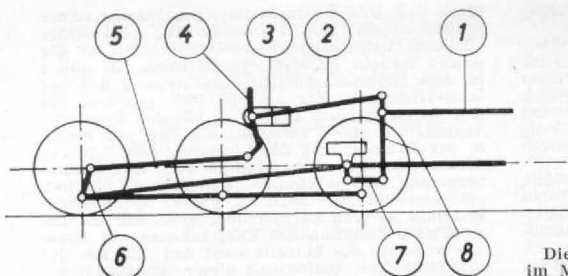
Abb. 4. Maßstäbliche Orientierungsskizze (M. 1:1) für den Triebwerksumbau. Die neuanzufertigenden Teile 1—8 entsprechen denen der Abb. 6.
