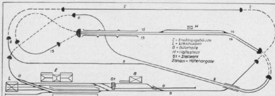
Streckenplan der H0-Anlage Hornbogen-Brust. Größe der Anlage 6,5 x 2 m, Maßstab ca. 1:150
