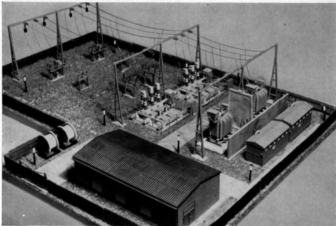
Abb. 1. Das hier abgebildete Modell entstand aus dem KIBRI-Bausatz 9925. Vor dem zweiten Abspanngerüst (von links gesehen) entdecken Sie eine sog. „Hilfsschiene“, die die beiden ersten Stromschiene verbindet, und die nur unter gewissen Umständen am Platze ist (daher fehlt sie auch im kleinen Bausatz 9924). Wir werden auf diese „Hilfsschiene“ im 2. Teil noch ausführlich eingehen, wollen jedoch bereits heute schon darauf hinweisen!
