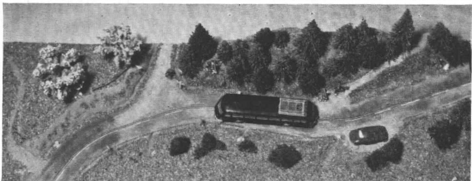
Abb. 4. Nicht mehr wiederzuerkennen sind die Straßenteile der Abb. 3, wenn sie – durch Verwendung abgesägter Teilstücke – richtig als Landstraße im Gelände verlegt und farblich getönt sind. Die feine Führungsrille ist kaum als solche zu erkennen. (Unretuschierte Archiv-Aufnahme!)
