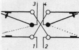
Abb. 2. Kontaktanordnung eines normalen zweipoligen Umschaltrelais.
