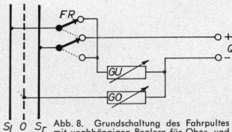
Abb. 8. Grundschialtung des Fahrpulses mit unabhängigen Reglern für Ober- und Unterleitung bei Vorwärtsfahrt.
