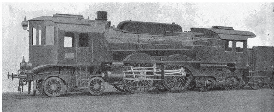
2 B 2-Schnellfahrlok der preuß. Staatsbahn, maximale Geschwindigkeit 137 km/h (1904).
