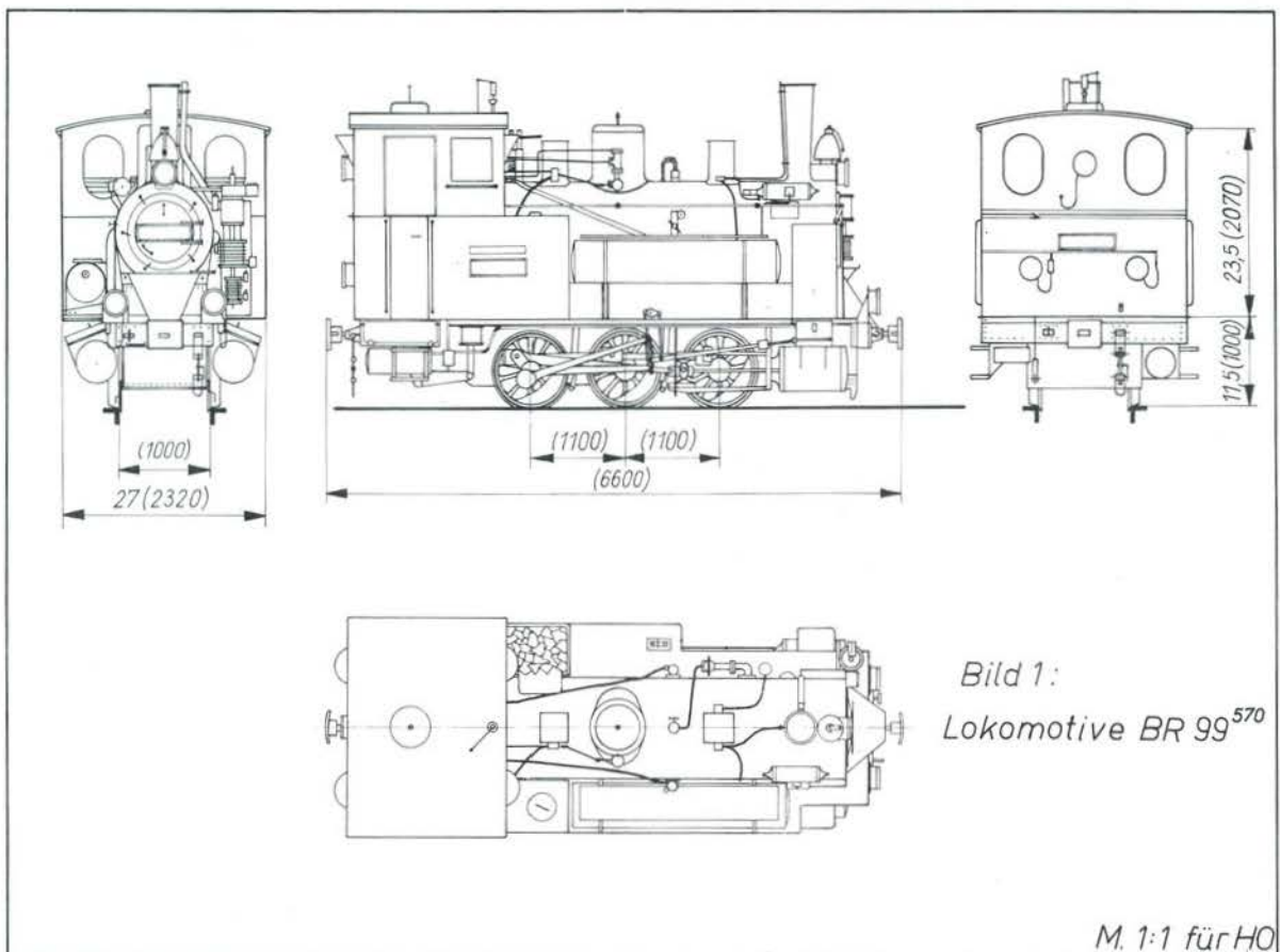
Bild 1 Maßbild
