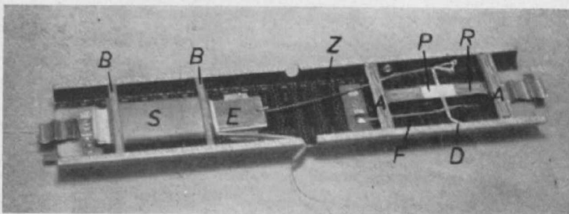
Abb. 6. Die fertige Entkupplungsvorrichtung in einem geraden Märklin-Gleisstück. Buchstabenerklärung siehe Text.
