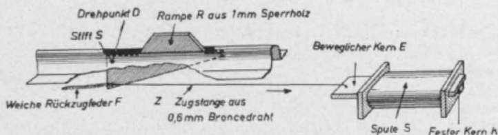
Abb. 7. Die elektromechanische EKV für ein Trix-Gleis (Stellung Entkupplungsrampe oben)
