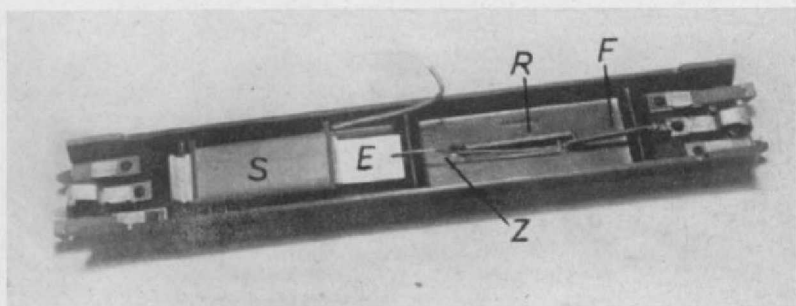
Abb. 8. Auch beim Trix-Gleis verschwindet der gesamte Mechanismus im Gleiskörper.
