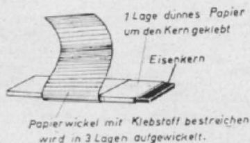
Abb. 5. So stellen wir den Magnetspulenkörper aus Papier und 1-mm-Sperrholz her.
