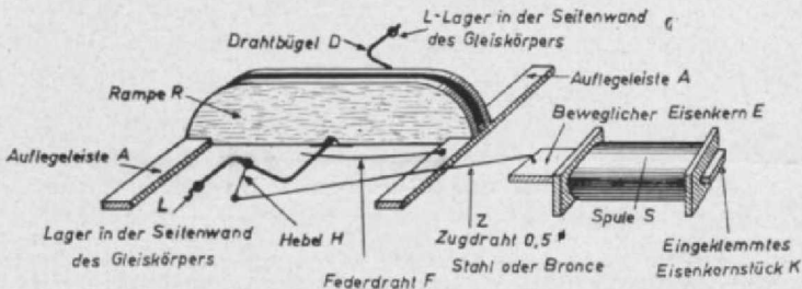
Abb. 2. Die elektromechanische Anordnung der EKV für Märklin-Gleise. Entkupplungsrampe in „Ruhestellung“ (also „unten“) gezeichnet.
