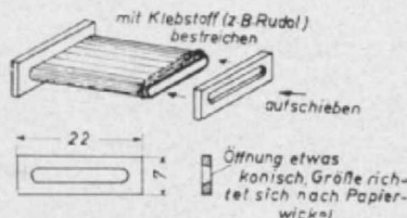
Abb. 5. So stellen wir den Magnetspulenkörper aus Papier und 1-mm-Sperrholz her.
