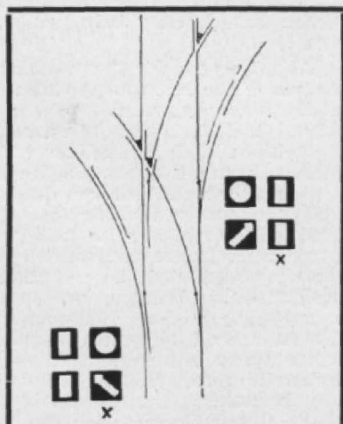
Abb. 2. Bei der symmetrischen Doppelweiche stehen die Weichenlaternen links und rechts. Signalbild bei Geradeaus-Stellung der Weiche angekreuzt
