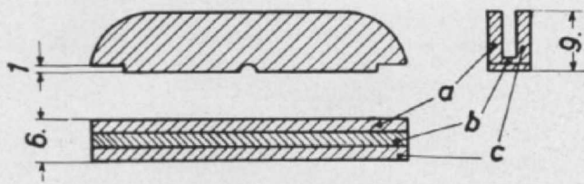
Abb. 3. Entkopplungsrampe für Märklin im Maßstab 1:1.
