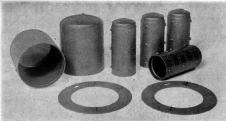
Abb. 8. Das sind einige der Einzelteile, aus denen die Hydrierürme zusammengesetzt werden. Ein „dünnerer“ Kessel kostet DM 0.45, der „dikke“ DM 0.60. Die Plattformen werden mit Geländer erhältlich sein. Ihr Preis: DM 0.30 und DM 0.40. Ein Sortiment Rohrleitungen verschiedener Stärke (Kunststoff) wird sich auf DM 0.90 stellen.
