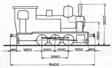
Abb. 18. Typenskizze einer „9921“ (K 33.6).
