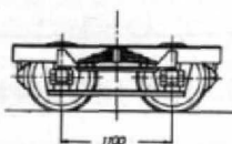
Abb. 7. Ein Drehgestell der HSA-Wagen in \frac{1}{2} H0-Größe (12-mm-Spur) zum Zweck des Selbstbaues.
