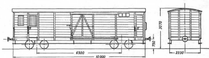
Abb. 1. Vierachsiger Gepäckwagen mit Postabteil der Kleinbahn Hoya-Syke-Asendorf (1000-mm-Spur).
