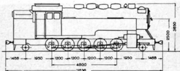
Abb. 14. Typenskizze der schweren DB-Schmalspurlok BR 99 22, Betriebsgattung K 57.10. Treibraddurchmesser 1000 mm, Laufreddurchmesser 550 mm, Spurweite 1000 mm. Größte Geschwindigkeit 40 km/h. Skizze in 1/2 H0-Größe. LÖP beträgt also in Baugröße H0 (Spur 12 mm) 13,5 cm. (Siehe auch „25 Jahre Deutsche Einheitslokomotive.“)
