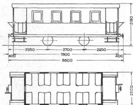
Abb. 10. → Schmalspur-personen-wagen der DB in 1/2 H0-Größe.
