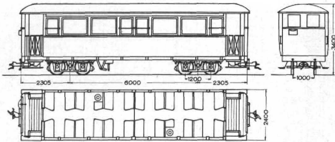
Abb. 8. Typenskizze eines modernisierten CC-Personenwagens der ebenfalls meterspurigen Oberrheinischen Eisenbahn (OEG) in \frac{1}{2} H0-Größe.
