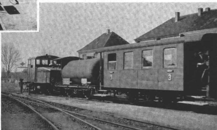
Abb. 12. Schmalspurzug bei der Ausfahrt aus Bahnhof Mundenheim. Zuglok V 29.
