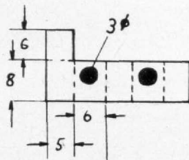
Abb. 6. Abwicklung des Laternenkästchens.
