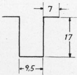
Abb. 6. Abwicklung des Laternenkästchens.
