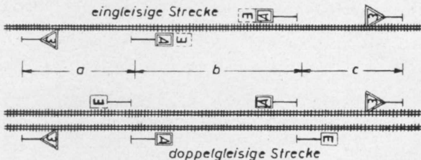
Abb. 2. So wird eine „Lafa“-Stelle beim Vorbild gekennzeichnet; die Zahl 3 bedeutet: 30 km/h.
