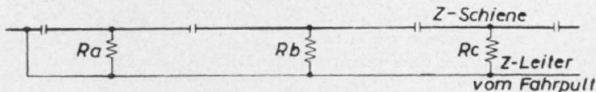
Abb. 3. Anschlußschema für die elektro-automatische Schaltung von „Lafa“-Strecken bei Modellbahnen für eine eingleisige Strecke. Bei doppelgleisigen Strecken sind die 3 Widerstände an jedem der beiden Gleise vorzusehen.
