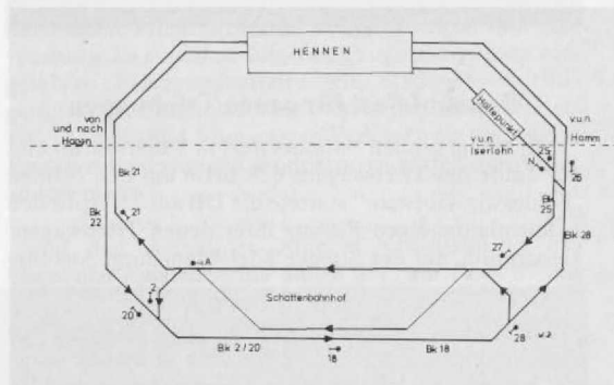
Bild 1. Block-Einteilung der Anlage
