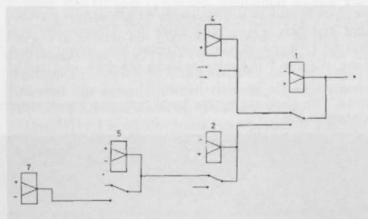
Bild 3. Prinzipskizze für Relais- und Weichenstellung.
