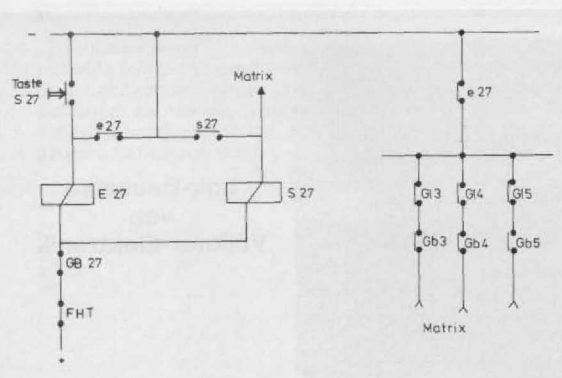
Bild 2. Schaltungsplan (siehe Haupttext).
