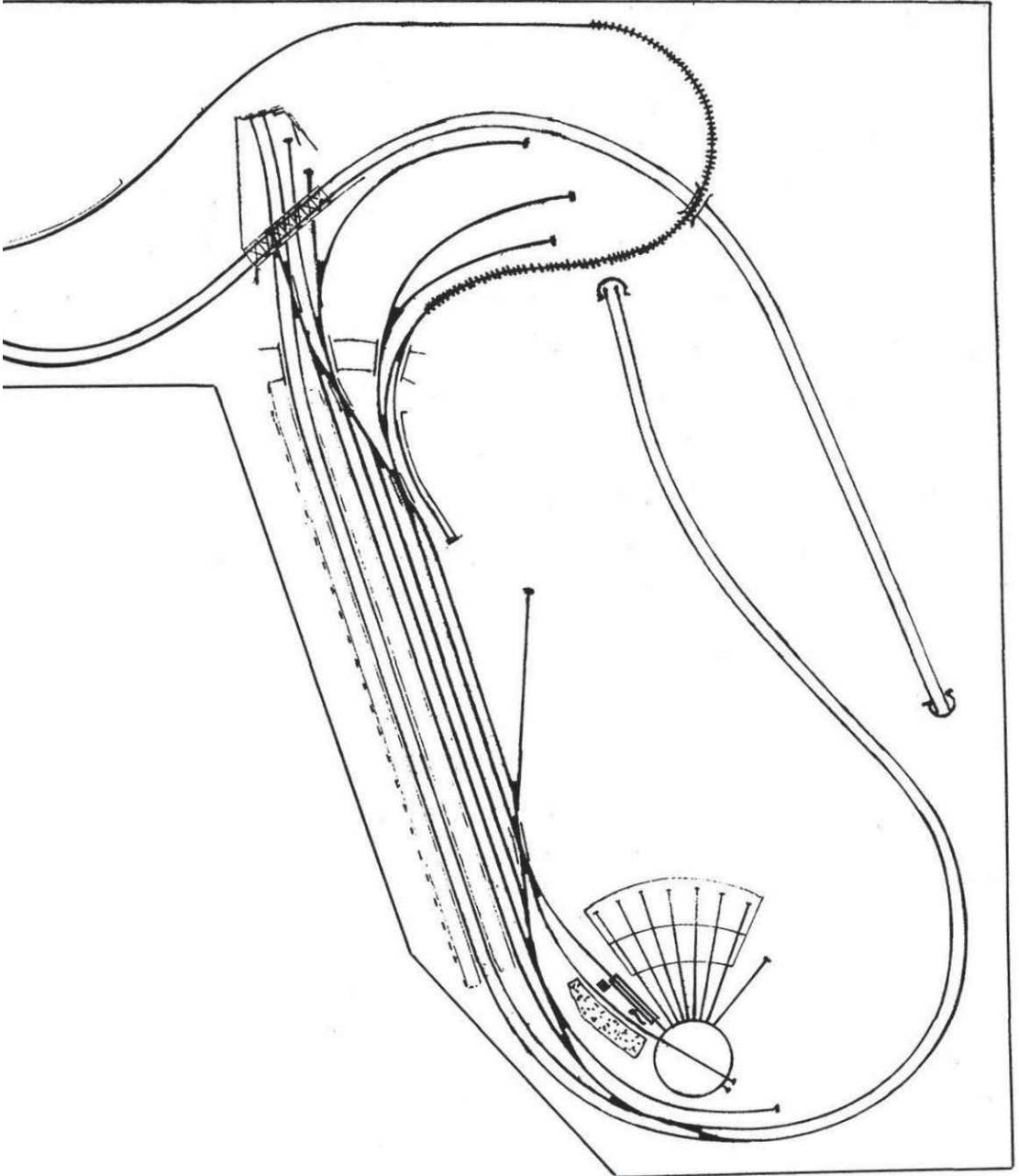
Die oberirdischen Gleisanlagen, wiedergegeben im Zeichnungsmaßstab 1:27. Die Zahnrad-Strecke ist gestrichelt dargestellt.
