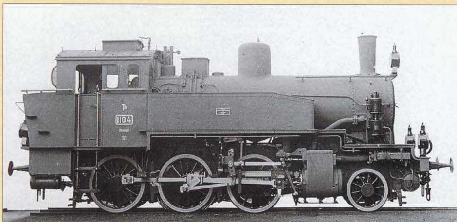
Bild 5: Auch die Kgl. Württ. Staatseisenbahnen beschafften zehn Lokomotiven dieses Typs nach preußischen Zeichnungen – hier die T 9 1104, die spätere 91 2004 der Deutschen Reichsbahn.
