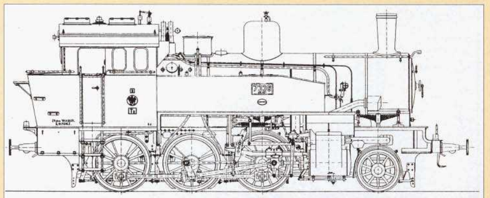
Bild 9: Typenzeichnung der preussischen T 9 3 im Maßstab 1: 87. Abb.: Sammlung Obermayer
