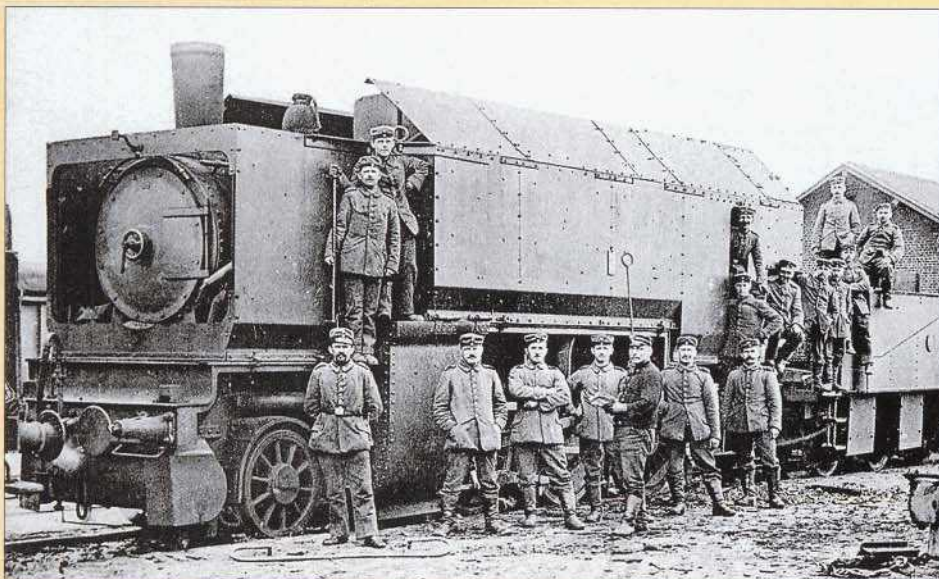
Bild 6: Eine T 9 3 als Panzerzuglokomotive, gekuppelt mit einem Tender als Wasserwagen. Abb. 4 bis 6: Sammlung Dr. Scheingraber
