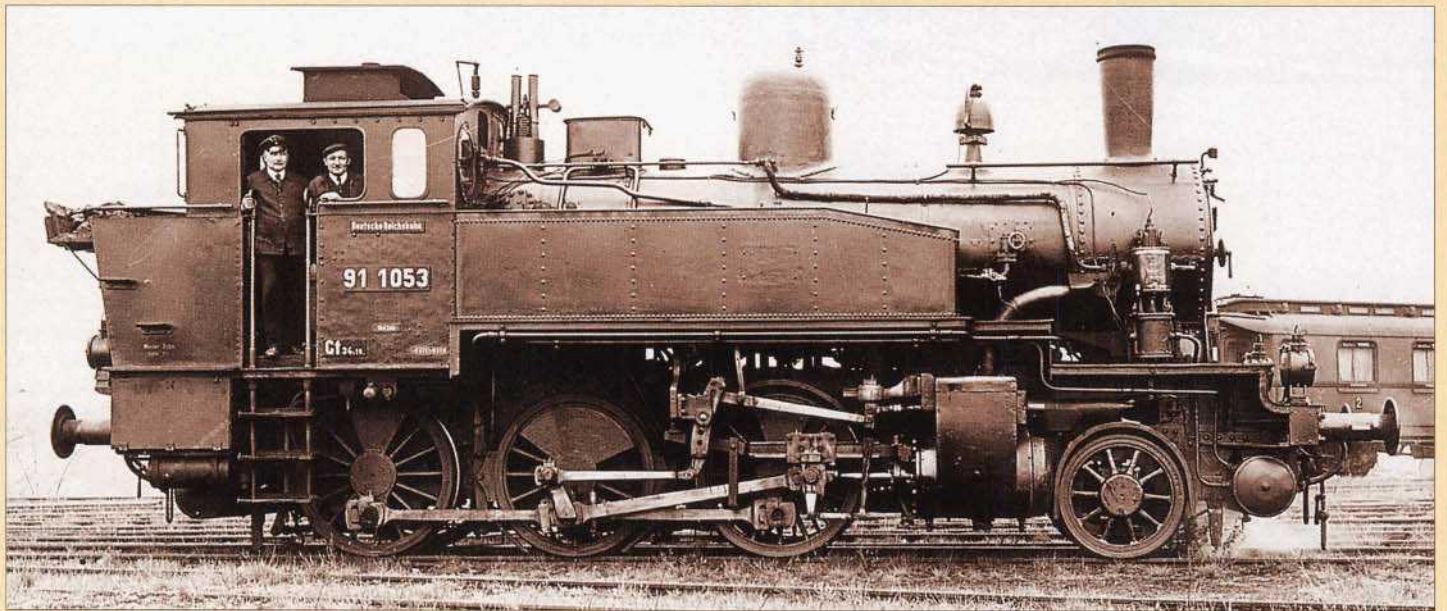
Bilder 7 und 8: Die beiden Aufnahmen verdeutlichen Unterschiede in der Bauausführung der T 9 3 . Abb. 7 und 8: Sammlung Obermayer
