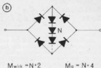
Abb. 3. Vergleich zwischen Anti-parallel- (a) und Brückenschaltung (b). M_g = Gesamtzahl der Dioden, M_{\text{wirk}} = Zahl der wirksamen Dioden. Bei M_{\text{wirk}} > 3 ist die Brückenschaltung weniger aufwendig.
