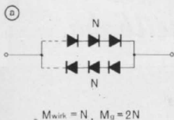
Abb. 3. Vergleich zwischen Anti-parallel- (a) und Brückenschaltung (b). M_g = Gesamtzahl der Dioden, M_{\text{wirk}} = Zahl der wirksamen Dioden. Bei M_{\text{wirk}} > 3 ist die Brückenschaltung weniger aufwendig.
