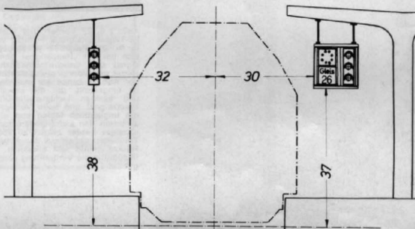
Abb. 5. Zwei weitere Lichtsignal-Bonbons aus dem NMW-Katalog (Wiedergabe in \frac{1}{4} Originalgröße): Bremsprobensignal solo (links) sowie kombiniert mit Abfahrtauftrag-Signal (Zp9) und Gleisnummerierung, hier in der Ausführung als Hängesignal. Es ist auch als Ausleger- oder Stand-signal erhältlich.
