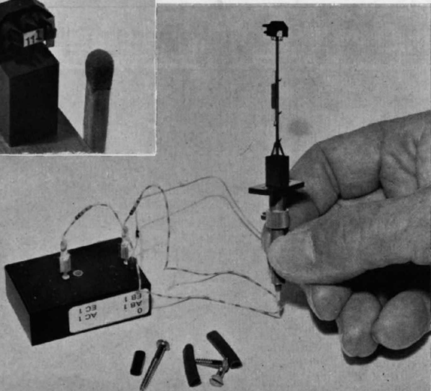
Abb. 9. Ein nicht minder exzellentes Gleissperrsignal in hoher Ausführung mit Einbausockel und Befestigungsring (s. Haupttext). Die Kabel führen zu dem Spannungsadapter, über den jedes Signal angeschlossen werden muß, da sonst unweigerlich die Optiken zerstört werden. Vor dem Adapter liegen farbige Kennzeichnungstüllen für die Anschlußkabel und Befestigungsschrauben; beides ist jedem Signal beigegeben.
