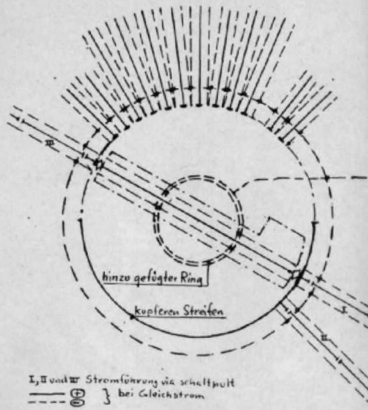
Abb. 4. Prinzipdarstellung des Stromverlaufs: Die vom Verfasser als „hinzugefügter Ring“ bezeichneten (ringförmigen) Kontaktstreifen aus Kupferblech dienen zur Fahrstrom-Rückleitung und zur Bühnenhaus-Beleuchtung; über die „kupfernen Streifen“ erfolgt die Zufuhr des Fahrstroms, dessen Rückleitung bei I, II und III über ein Schaltpult (zum Abschalten einzelner Gleisabschnitte). Die Angaben „+“ und „-“ beziehen sich auf das vom Erbauer verwendete Dreischienen-Gleichstrom-System.
