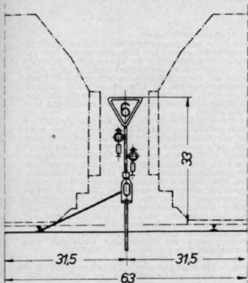
▼ Abb. 8. Das Zwergsignal nochmals in vergrößerter Wiedergabe, um u. a. die vorbildgetreu unsymmetrische Form der Schuten über den Lichtaustritts-Öffnungen zu zeigen, durch die im Großen Fremdlichteinfall verhindert werden soll.
