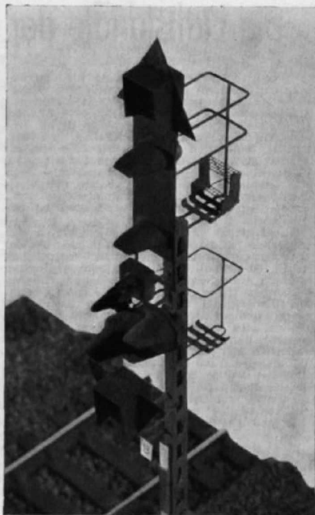
Abb. 3 u. 4. Zwei Nahansichten des Signals der Abb. 1 u. 2 (in ca. doppelter Originalgröße), die für sich bzw. die überdurchschnittlich exakte und filigrane Ausführung sprechen dürften! Die selbstklebenden Signal-Bezeichnungen (hier z. B. das „B“) stammen von einem Ausschneidebogen, der extra erhältlich ist.
