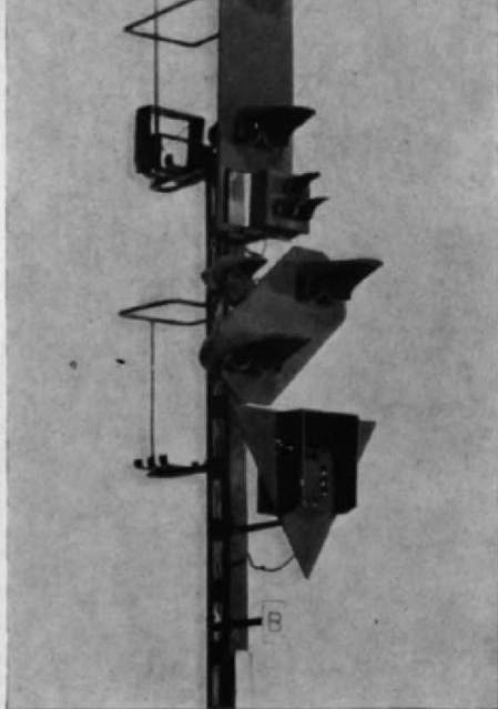
Abb. 3 u. 4. Zwei Nahansichten des Signals der Abb. 1 u. 2 (in ca. doppelter Originalgröße), die für sich bzw. die überdurchschnittlich exakte und filigrane Ausführung sprechen dürften! Die selbstklebenden Signal-Bezeichnungen (hier z. B. das „B“) stammen von einem Ausschneidebogen, der extra erhältlich ist.
