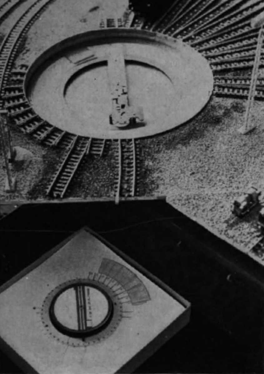
Abb. 3. Die Steuerung der umgebauten Drehscheibe erfolgt mit dem Original-Arnold-Schalter.
