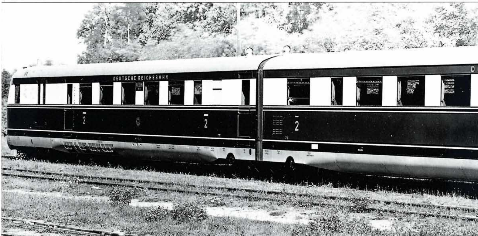
Bild 19: SVT 137 229 im August 1935 in Görlitz vor der Ablieferung. Abb.: WUMAG, Slg. Dietz
