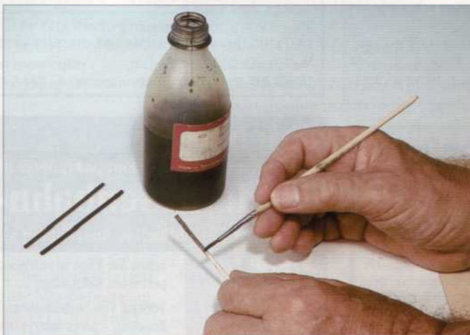
72 Geradezu ein Wahrzeichen der „guten alten Eisenbahn“ waren die Telegrafleitungen, die die Bahnstrecken über viele Kilometer begleiteten. Wie man die entsprechenden Masten in H0 herstellt, beschreibt unser Beitrag. Foto: Thomas Mauer
