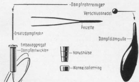
Abb. 2. Aus diesen Teilen besteht der komplette Satz, während das Einbauaggregat selbst lediglich aus dem Dampfentwickler, der Konushülse und der Wärmeisolerierbuchse besteht.
