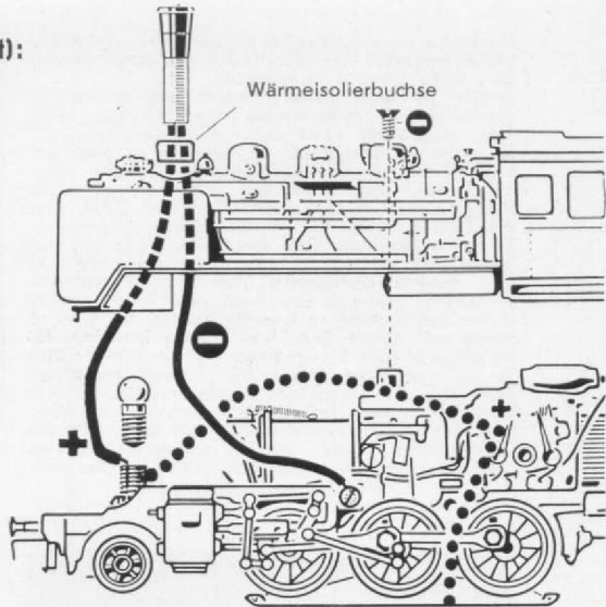
Abb. 1. Der Einbau des Dampfentwicklers in eine Märklin-Lok. Die —Leitung (braunes Kabel) ist Massepol.
