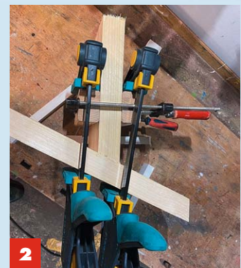
2 Verbindungsstellen mit Dübeln und Leim verbinden. Mit noch zwei Zwingen fixieren.
